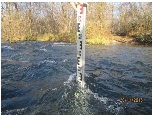
Foto 9 - Altezza d'acqua misurata in centro alveo
